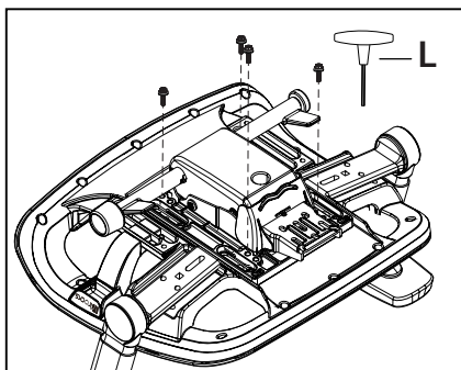
▲ 圖為底盤螺絲拆卸處
