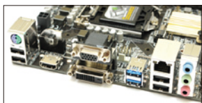
● 背板提供HDMI、DVI、D-Sub三種顯示輸出。
